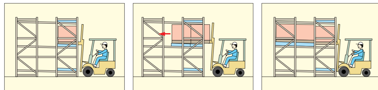
A 収納物を台車に載せます。 B 最初の収納物を押し込みながら次の台車に収納物を載せます。 C 収納物を押し込みながら最後はレールの上に収納物を載せます。
