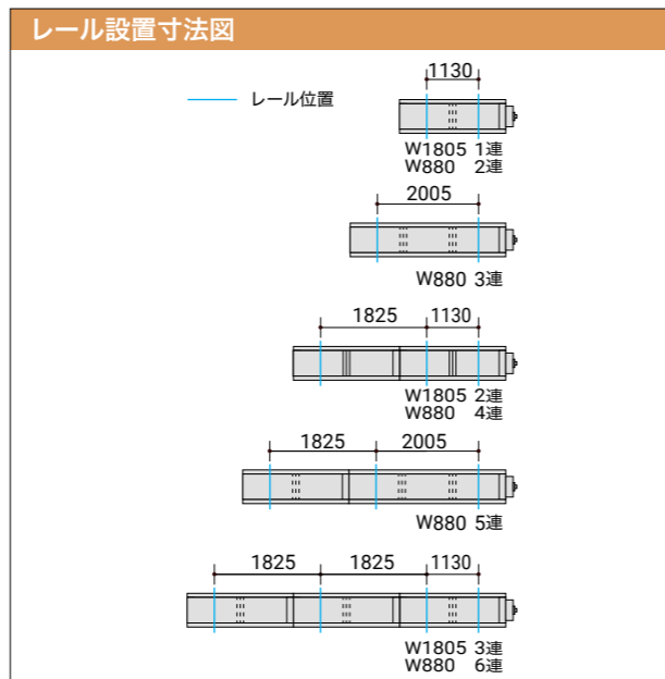
※レール設置寸法は、レール中心線を基準としています。
